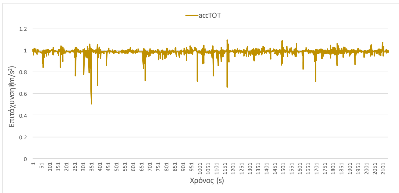
Διάγραμμα 3.5 Μετρήσεις επιταχυνσιόμετρου ίδιου ταξιδιού με αυτοκίνητο με τη χρήση της συνισταμένης
