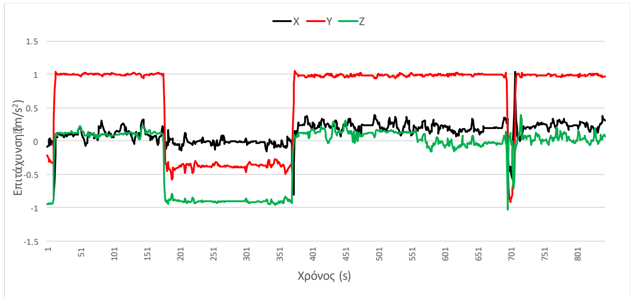
Διάγραμμα 3.2 Μετρήσεις επιταχυνσιόμετρον ενός ταξιδιού με τα MMM με τη χρήση 3 αξόνων
