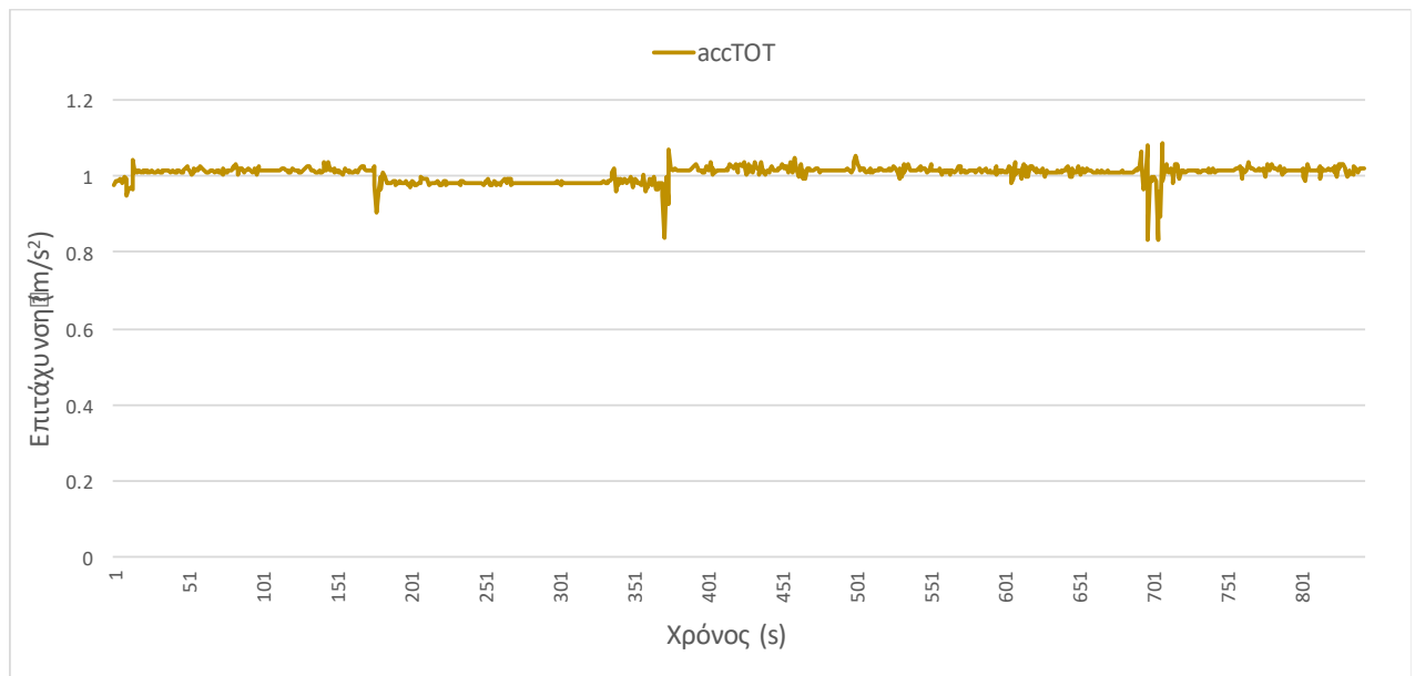
Διάγραμμα 3.3 Μετρήσεις επιταχυνσιόμετρον ίδιου ταξιδιού με τα MMM με τη χρήση της συνισταμένης
