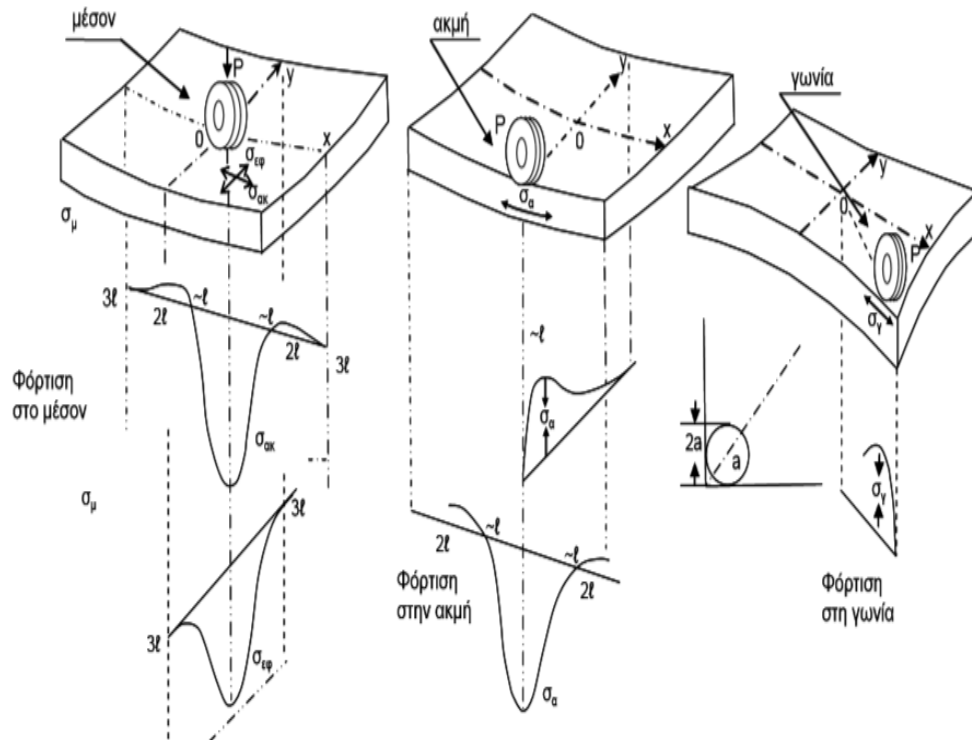
Σχήμα 2.1: Αναπτυσσόμενες τάσεις σε πλάκα από σκυρόδεμα κατά Westergaard
