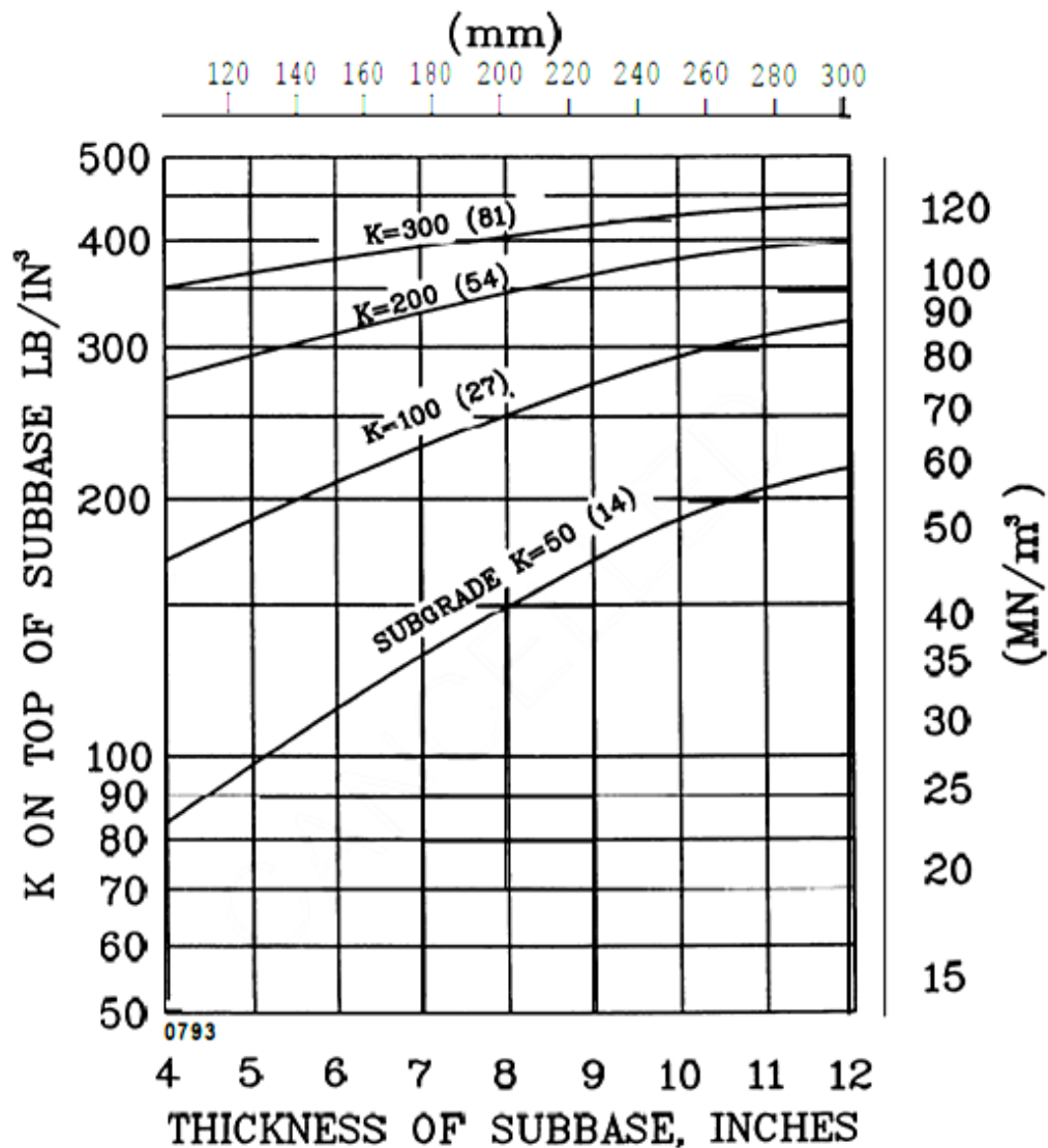
Σχήμα 2.9: Υπολογισμός K στην επιφάνεια της υπόβασης από ασύνδετο υλικό
