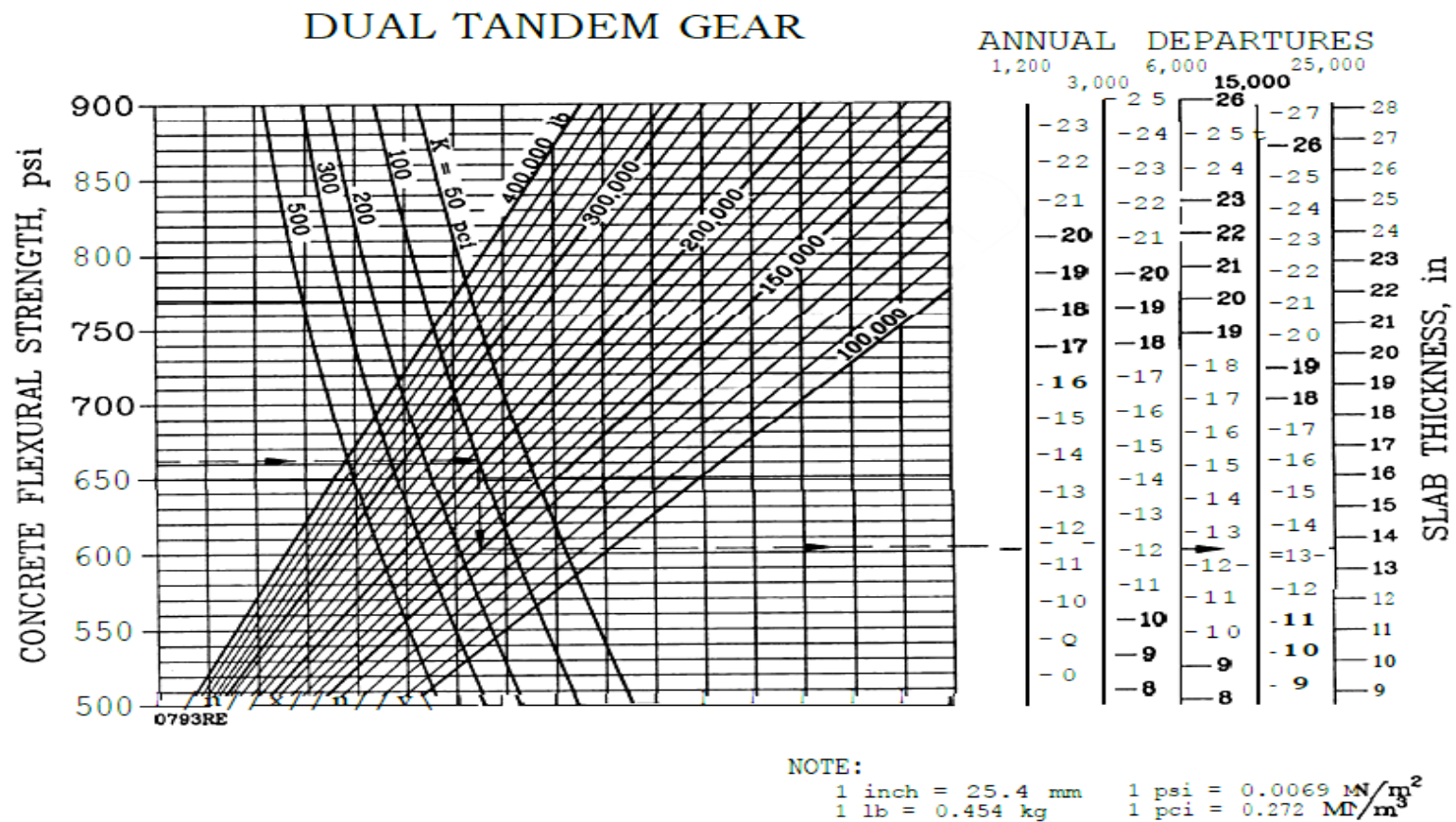
Σχήμα 2.13: Διάγραμμα υπολογισμού δύσκαμπτου οδοστρώματος για τυπικό φορείο διπλού τροχού διπλού άξονα (σειρά 2: δάπεδα στάθμευσης - δάπεδα αναμονής)
