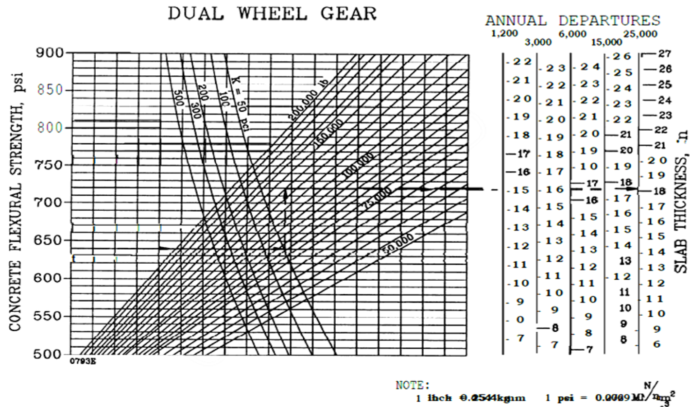
Σχήμα 2.11: Διάγραμμα υπολογισμού δύσκαμπτου οδοστρώματος για τυπικό φορείο διπλού τροχού (σειρά 1&2)
