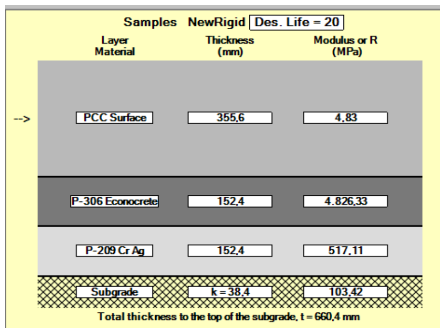
Σχήμα 3.15: Επιφάνεια εργασίας λογισμικού FAARFIELD
