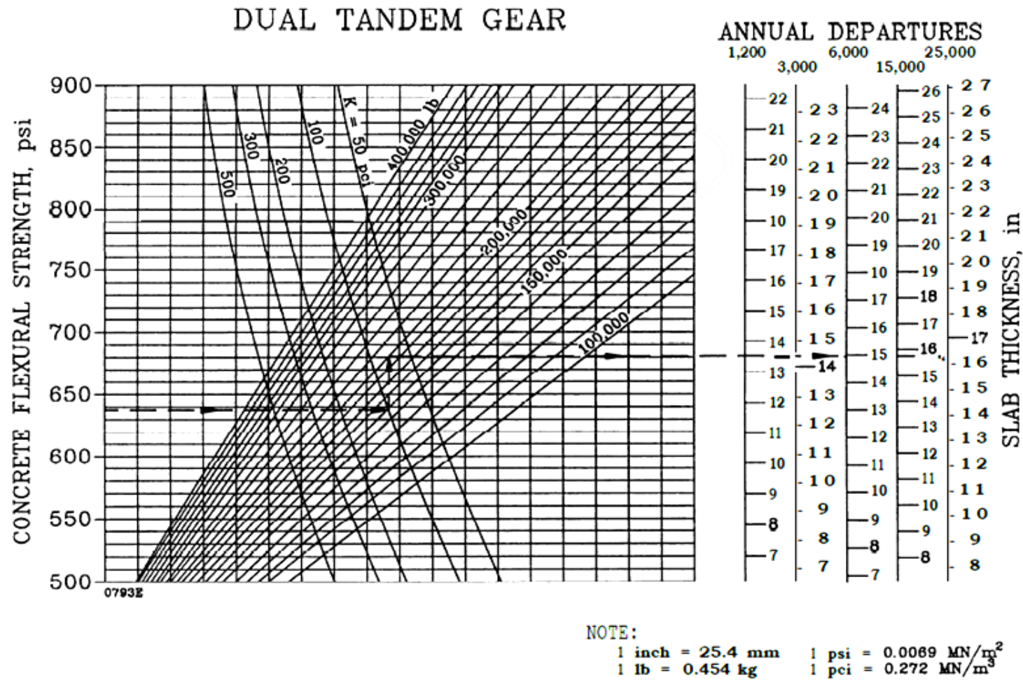
Σχήμα 2.12: Διάγραμμα υπολογισμού δύσκαμπτου οδοστρώματος για τυπικό φορείο διπλού τροχού διπλού άξονα (σειρά 1: διάδρομοι-τροχόδρομοι)
