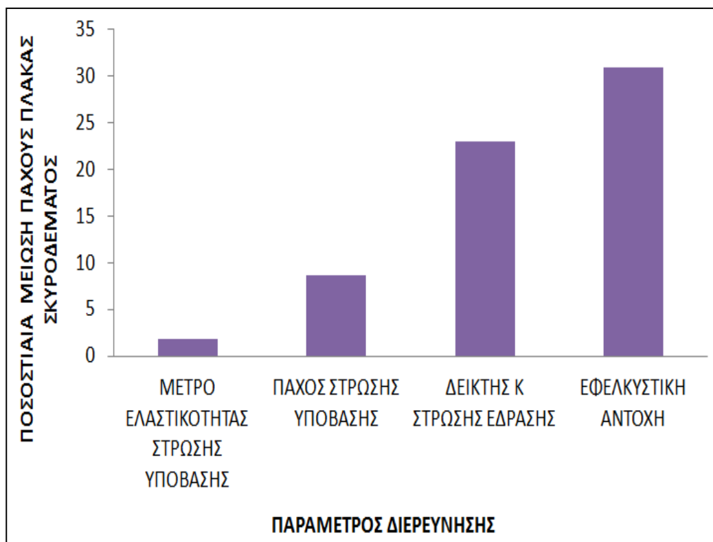
Σχήμα 5.10: Ποσοστιαία μείωση πάχους πλάκας σκυροδέματος για κάθε παράμετρο διερεύνησης
