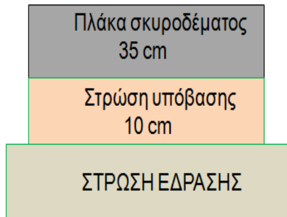
Σχήμα 5.23: Διατομή διερεύνησης για την επίδραση της μεταβολής του δείκτη αντίδρασης Κ στρώσης έδρασης στο δείκτη αθροιστικής φθοράς
