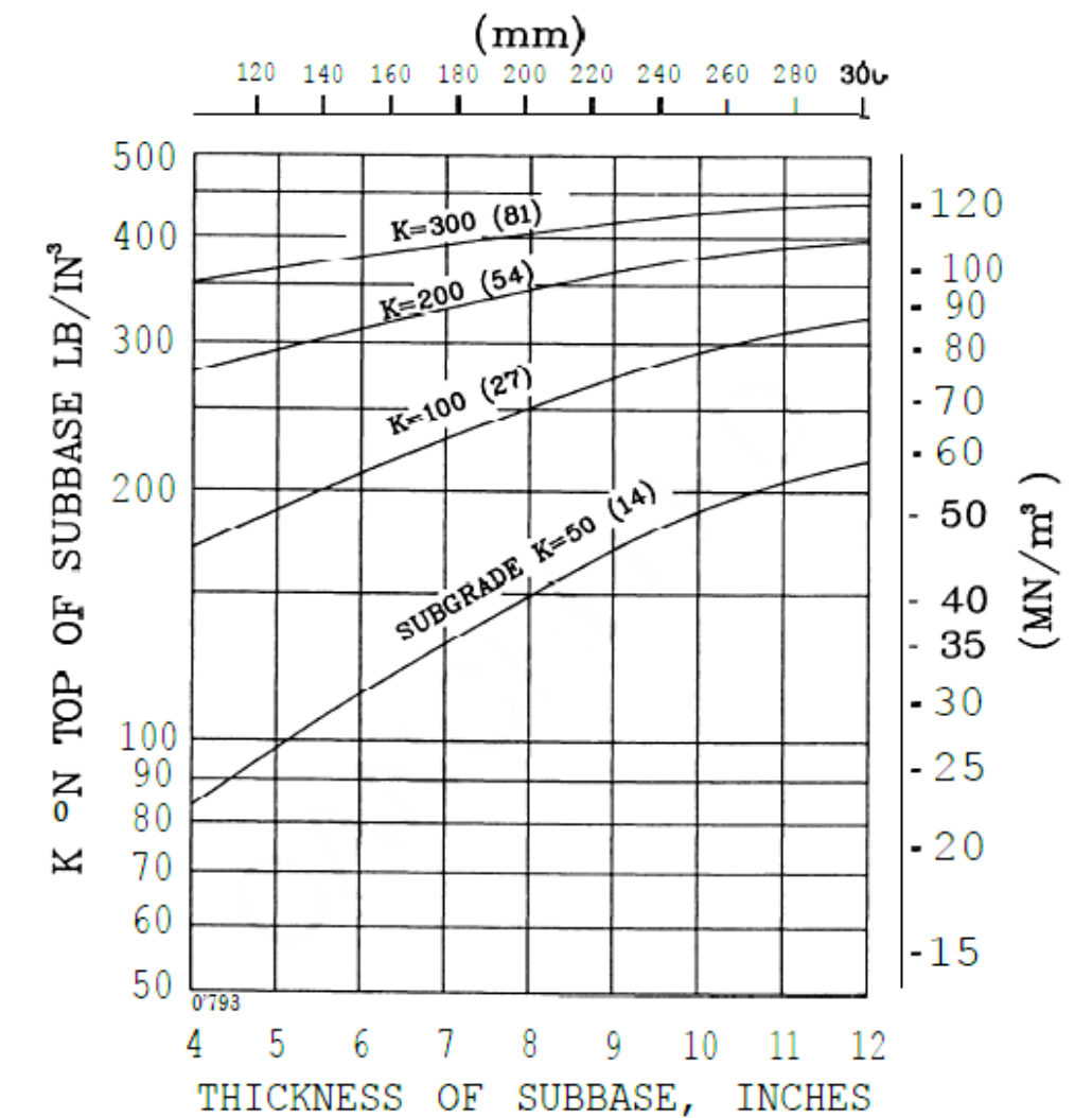
Σχήμα 2.8: Υπολογισμός K στην επιφάνεια υπόβασης από σταθεροποιημένα υλικά
