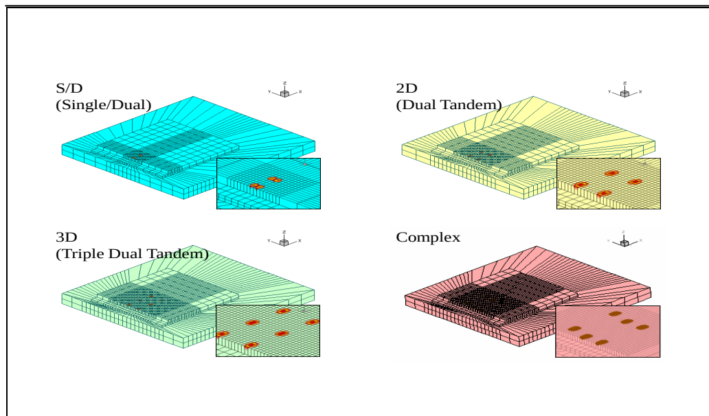
Σχήμα 3.3: Προσομοίωση συστημάτων τροχών αεροσκαφών με τη μέθοδο πετρερασμένων στοιχείων
