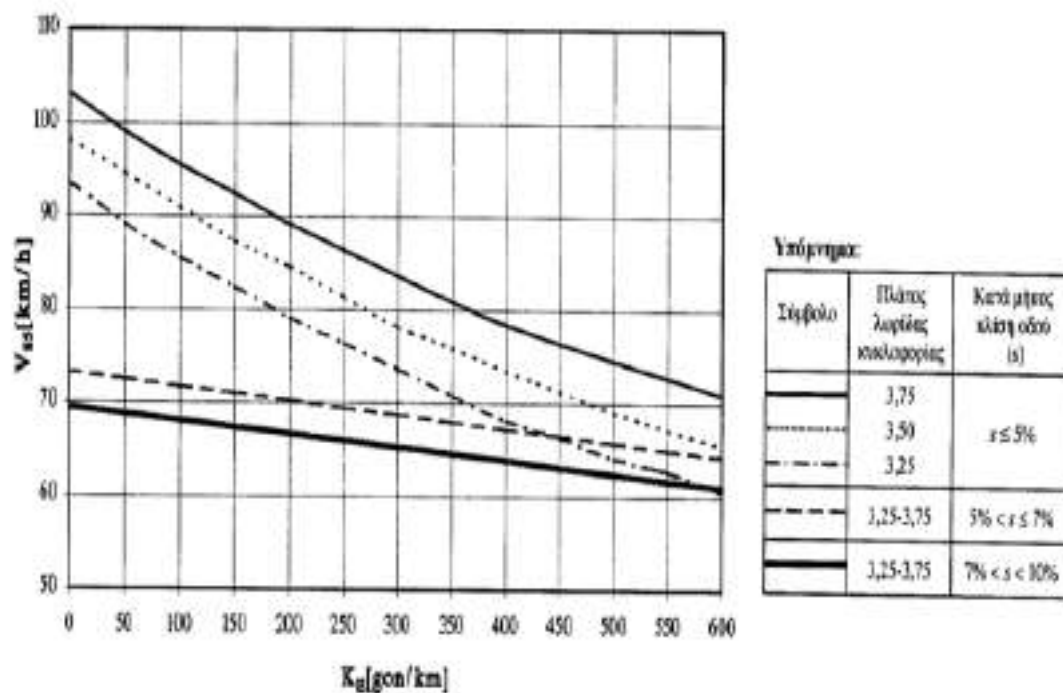
Σχήμα 27. Διάγραμμα υπολογισμού της λειτουργικής ταχύτητας V85 σε συνάρτηση με την ελκτικότητα (το τεταμένο) KE της μεμονωμένης καμπύλης και το πλάτος της λωρίδας κυκλοφορίας b σε υπεραστικές οδούς με ενιαία επιφάνεια κυκλοφορίας κατηγορίας ΑΙ έως ΑΙV (ΟΜΟΕ 2001b)
