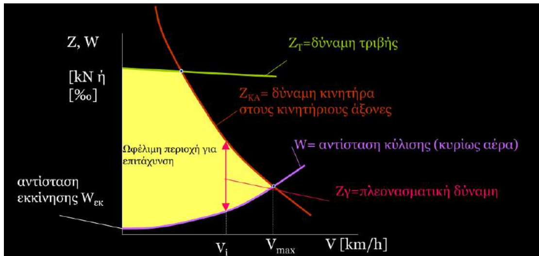
Εικόνα 16: Διάγραμμα Έλξης Κωνσταντίνου Λυμπέρη [25]
