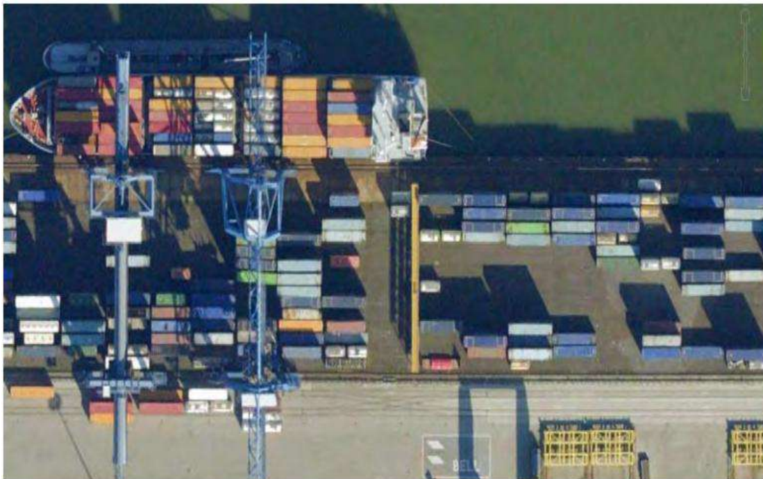
Εικόνα 53: Πλοίο εσωτερικής ναυσιπλοΐας με εμπορευματοκιβώτια των 45 ποδών στον λιμένα του Ρότερνταμ
