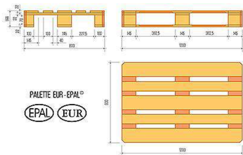
Εικόνα 57: Ευρωπαϊλέτα
