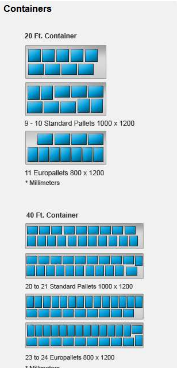
Εικόνα 58: τα κοντέινερ 20 και 40 ποδιών (εξωτερικό πλάτος 2,44 μέτρα)
