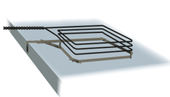
Εικόνες 4.10 και 4.11: Απλός επαγωγικός βρόχος σε σχεδιαστική απεικόνιση (αριστερά) και μετά την εγκατάσταση (δεξιά)
