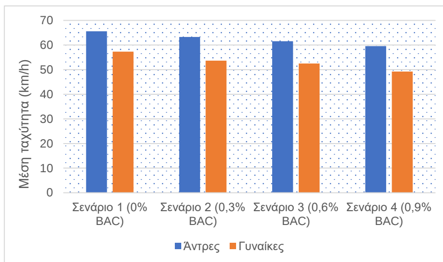
Γράφημα 4.6: : Μέση ταχύτητα ανά ποσότητα αλκοόλ ανά φύλο (km/h)
