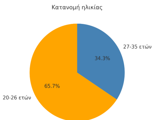
Γράφημα 4.2: κατανομή βάσει της ηλικίας
