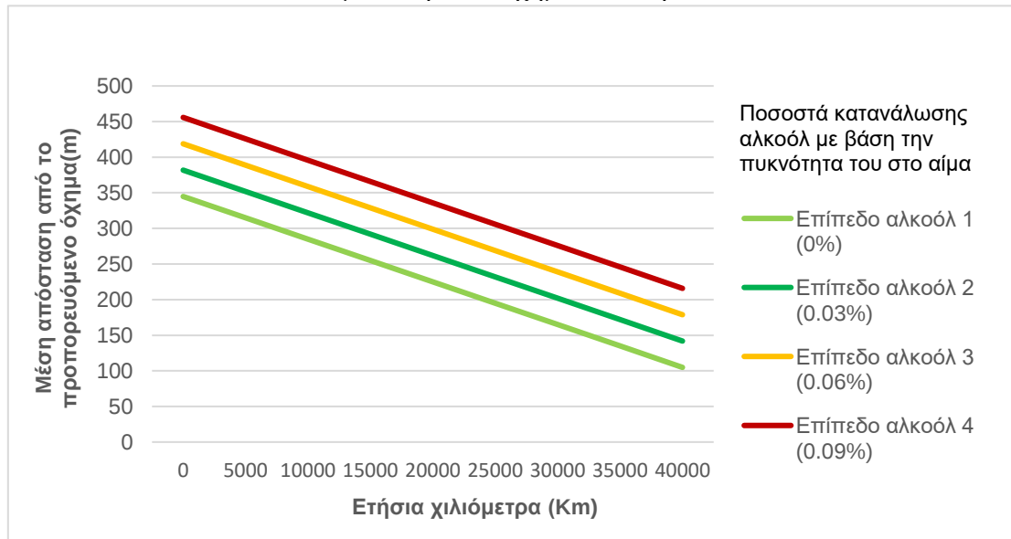
Διάγραμμα 5.7: Επίρροή των ετήσιων χιλιομέτρων που διανύει ο οδηγός που έχει εμπλακεί σε ατύχημα στο παρελθόν, στη μέση απόσταση από το προπορευόμενο όχημα.
