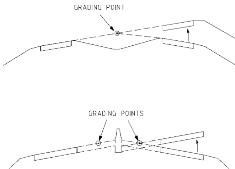
Σχήμα 2-13. Περιστροφή του οδοστρώματος για αστικές οδούς με διαχωρισμένα οδοστρώματα κατά AUSTROADS, 2021. [9]
