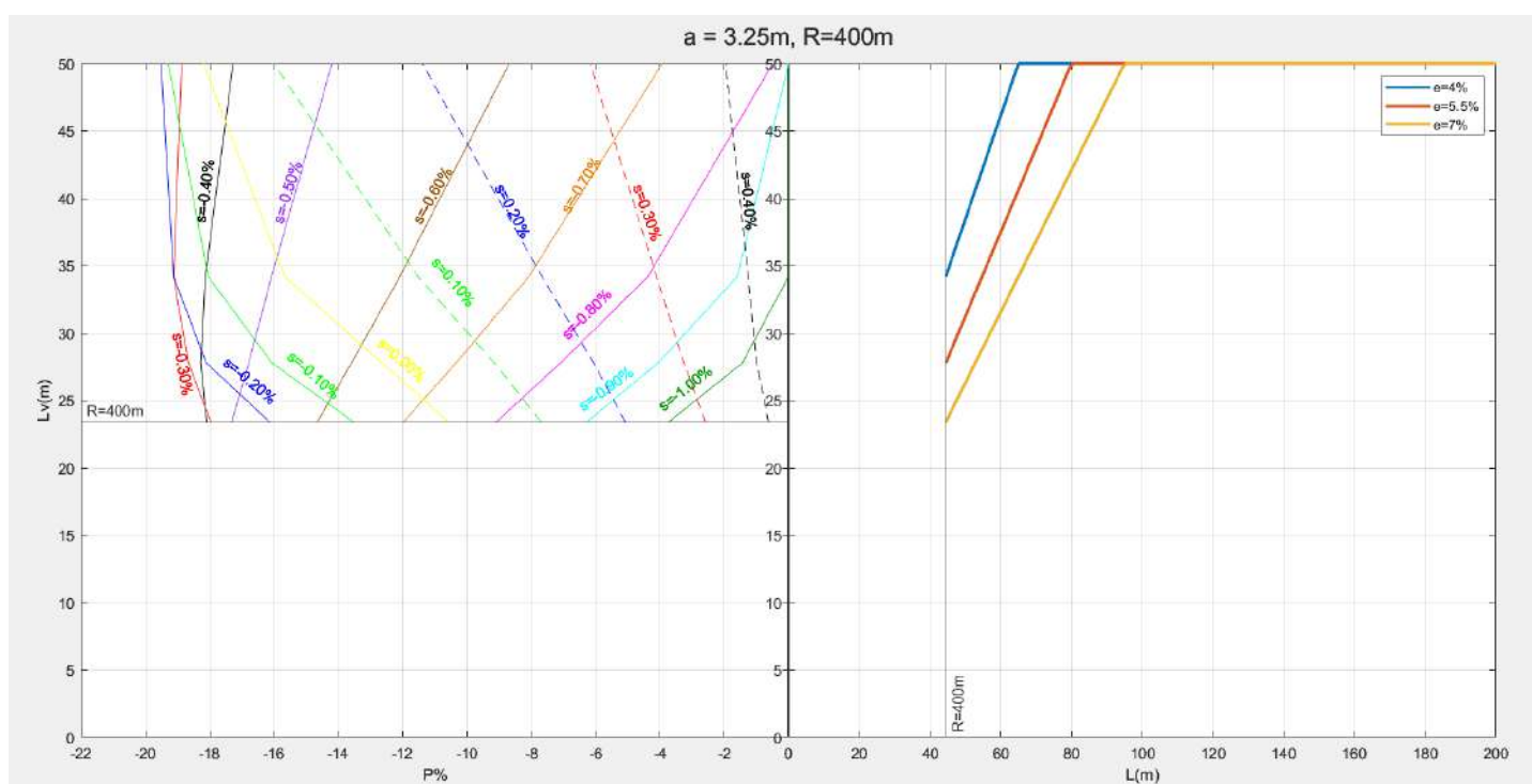
Σχήμα 5-2. Διάγραμμα εύρεσης ποσοστού των τιμών της σύνθετης κλίσης όπου p \leq 0.5\% , για \alpha = 3.25m και R = 400m .
