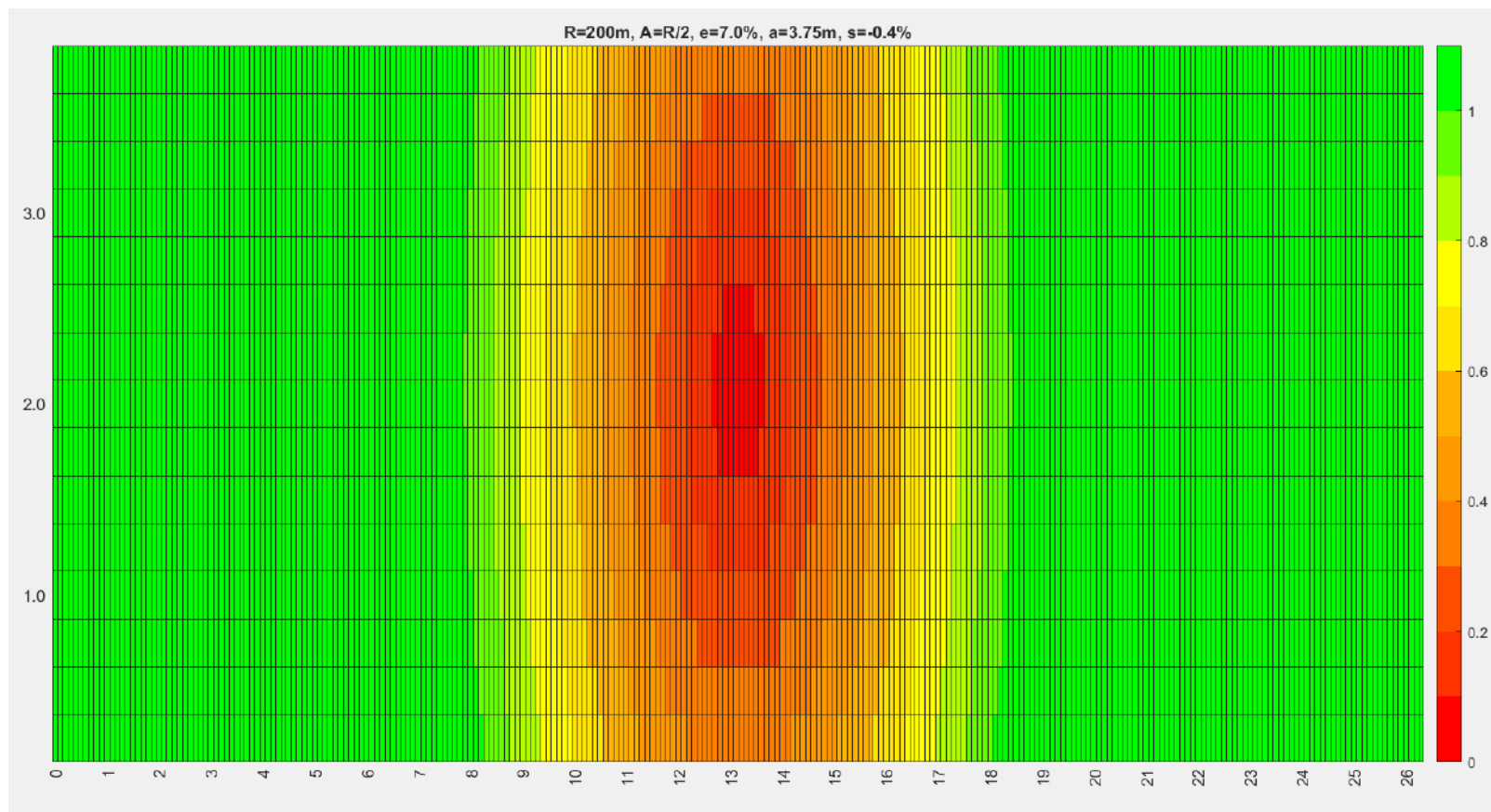
Π 12. Επιφάνεια ασθενούς απορρόγης ομβρίων για R=200m , A=R/2 , e=7\% , s=-0.4\% και a=3.75m .
