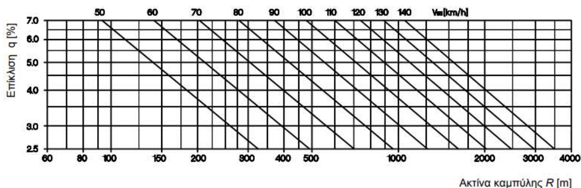
Σχήμα 2-16. Διάγραμμα προσδιορισμού της επίκλισης σε καμπύλες υπεραστικών οδών ΟΜΑΔΑ ΟΔΩΝ Α – ΛΟΦΩΔΗ ΚΑΙ ΟΡΕΙΝΑ ΕΔΑΦΗ, ΟΜΟΕ-Χ, 2001. [10]
