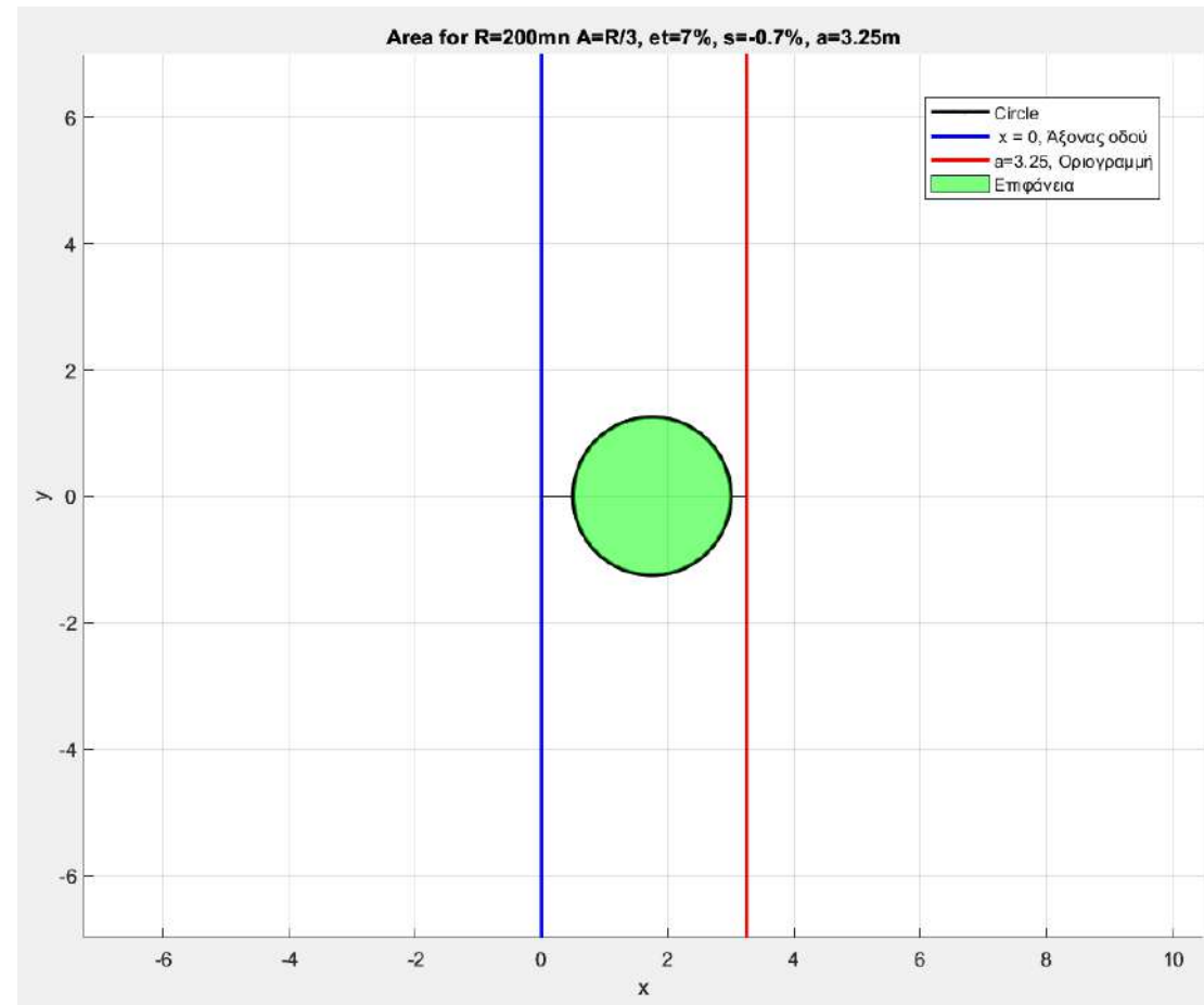
Π 1. Επιφάνεια ασθενούς απορροής ομβρίων για R=200\text{m} , A=R/3 , e=7\% , s=-0.7\% και a=3.25\text{m} .
