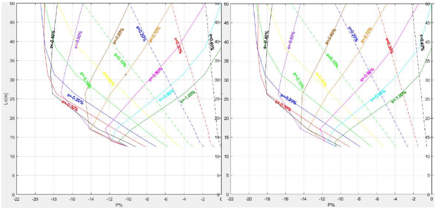
Σχήμα 5-1. Σύγκριση των 2 διαγραμμάτων για ποσοστά που προέκυψαν από την πρώτη μέθοδο (αριστερά) με αυτά που προέκυψαν από την δεύτερη (δεξιά) για \alpha = 3.75\text{m} .
