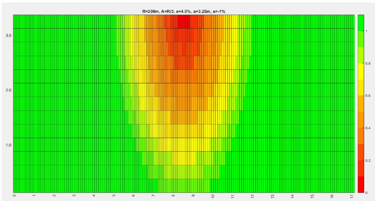
Π 9. Επιφάνεια ασθενούς απορροής ομβρίων για R=200m , A=R/3 , e=4\% , s=-1\% και a=3.25m .
