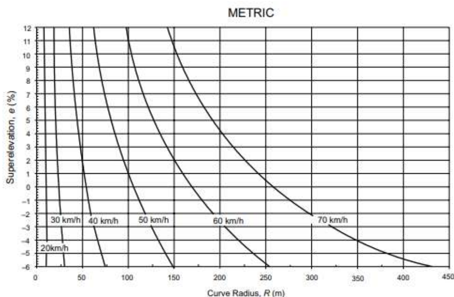
Σχήμα 2-6. Διάγραμμα προσδιορισμού της επίκλισης σε κυκλικά τμήματα, για αστικές περιοχές με χαμηλές ταχύτητες σχεδιασμού κατά AASHTO, 2018. [7]
