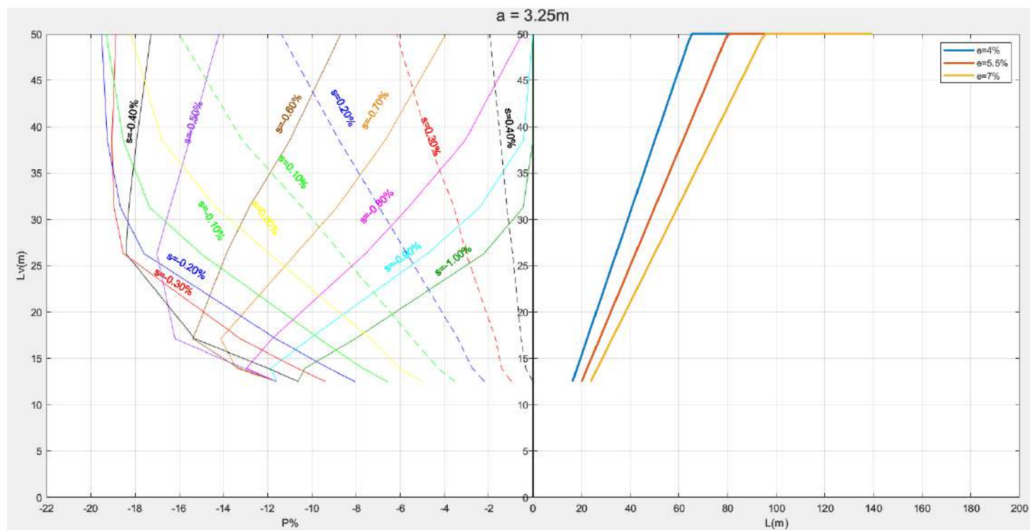
Σχήμα 4-6. Τελικό διάγραμμα υπολογισμού του ποσοστού όπου p \leq 0.5\% , για \alpha = 3.25m .
