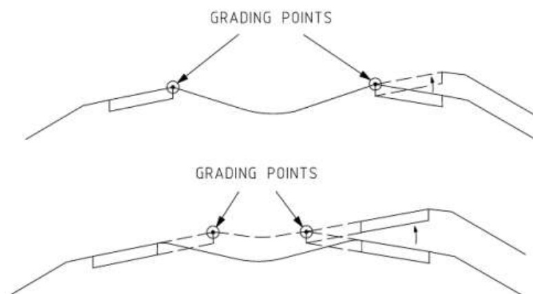
Σχήμα 2-14. Περιστροφή του οδοστρώματος για υπεραστικές οδούς με διαχωρισμένα οδοστρώματα κατά AUSTROADS, 2021. [9]
