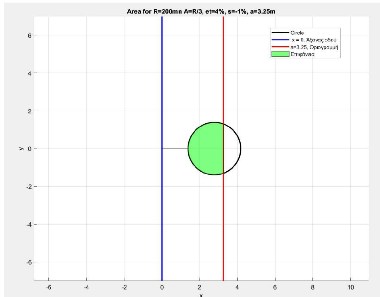
Π 2. Επιφάνεια ασθενούς απορροής ομβρίων για R=200m , A=R/3 , e=7\% , s=-1\% και a=3.25m .
