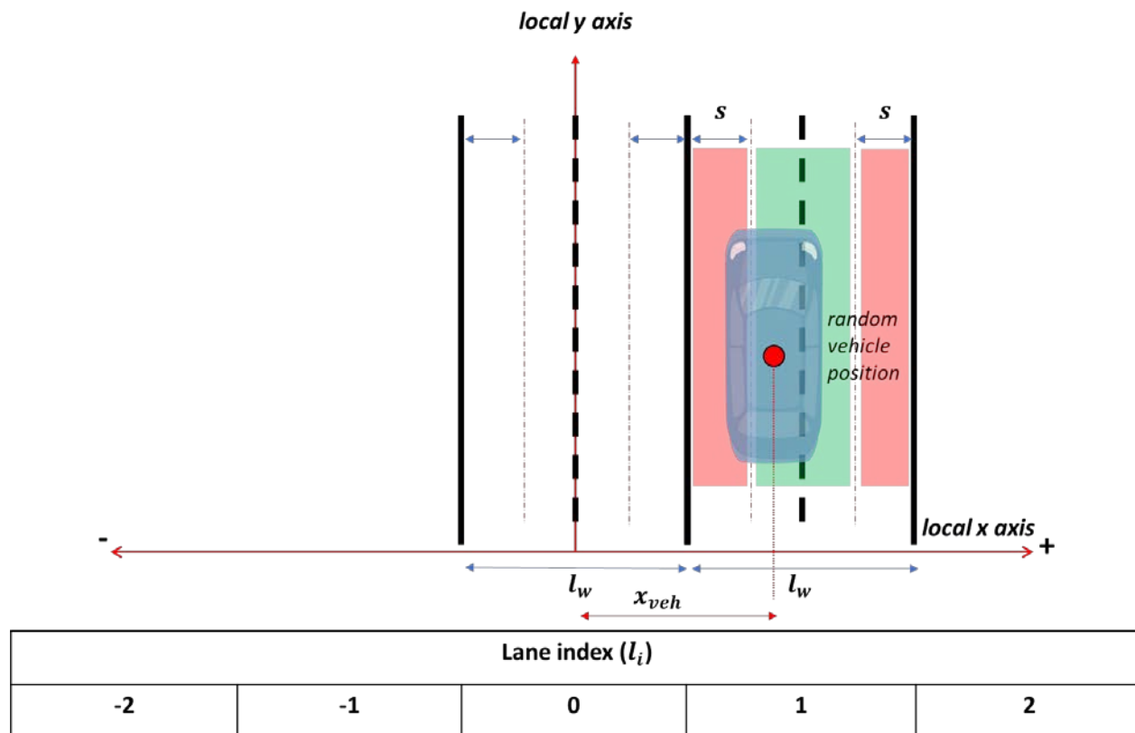
Σχήμα 4.2-8 Λογική εύρεσης της θέσης στις υπόλοιπες λωρίδες (αν αυτές υπάρχουν)
