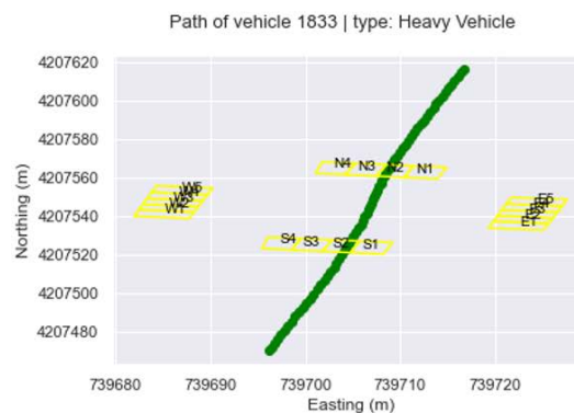
Εικόνα 4.2-18 Περίπτωση αξιοποιήσιμης και μη αξιοποιήσιμης πορείας οχήματος
