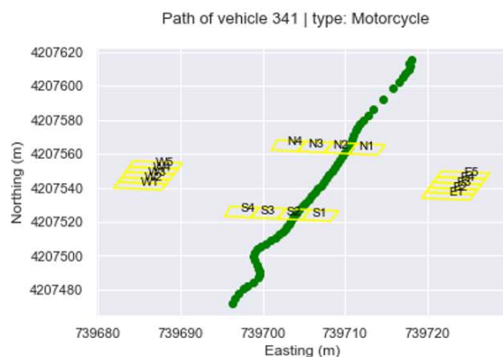
Εικόνα 4.2-18 Περίπτωση αξιοποιήσιμης και μη αξιοποιήσιμης πορείας οχήματος
