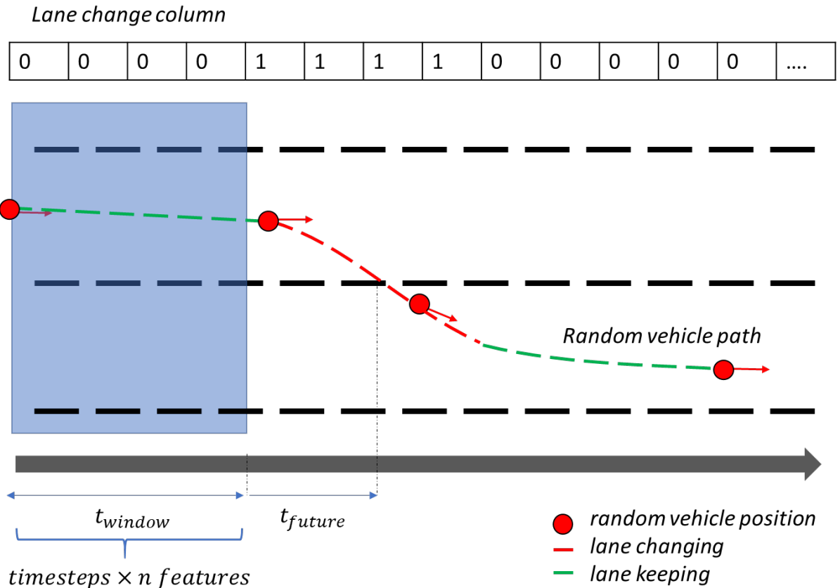
Σχήμα 4.4-1 Απεικόνιση του παραθύρου πρόβλεψης
