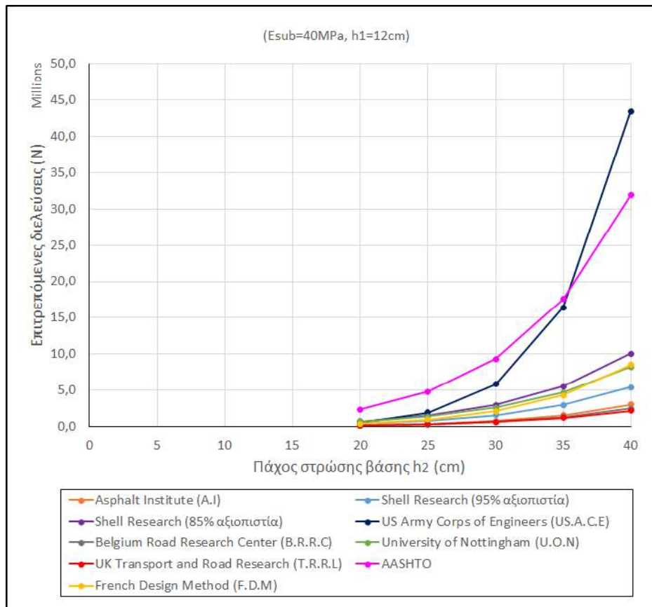
Εικόνα 4.18 Αποτελέσματα επιτρεπόμενων διελεύσεων N για μεταβολή του πάχους στρώσης βάσης και h_1=12\text{cm} & E_{\text{sub}}=40\text{MPa}
