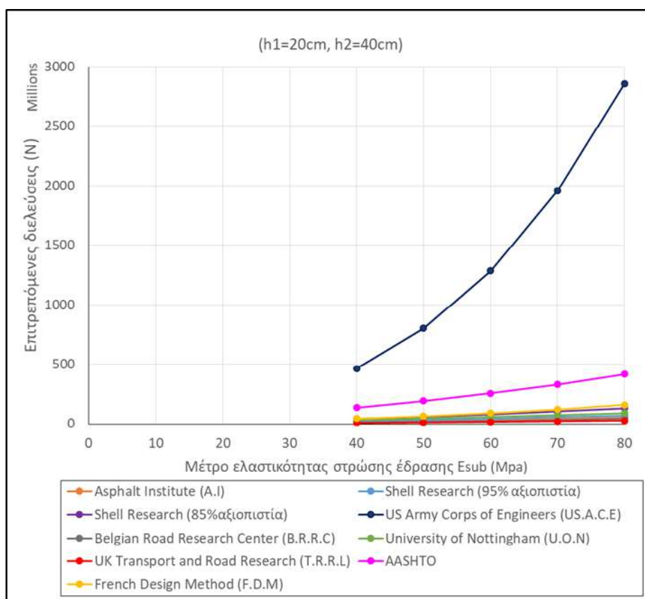
Εικόνα 4.26 Αποτελέσματα επιτρεπόμενων διελεύσεων N για μεταβολή του μέτρο ελαστικότητας E_{sub} και h_1=20\text{cm} & h_2=40\text{cm}
