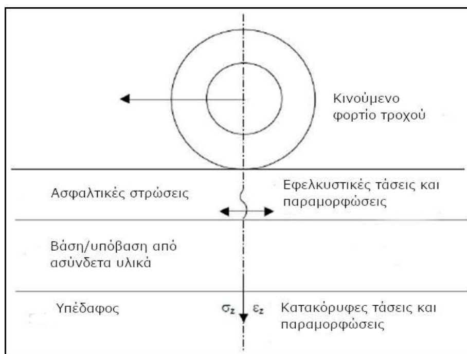
Εικόνα 3.1 Κρίσιμες θέσεις αστοχίας ενός εύκαμπτου οδοστρώματος (Acikgöz and Rauf 2010)
