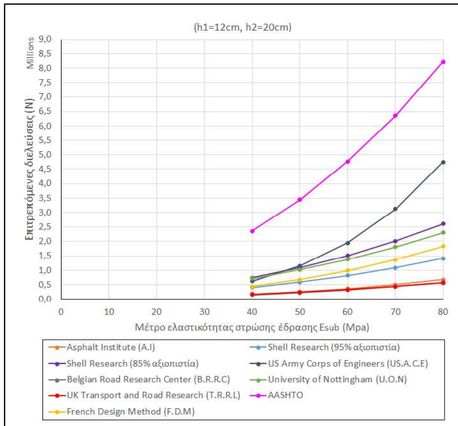
Εικόνα 4.24 Αποτελέσματα επιτρεπόμενων διελεύσεων N για μεταβολή του μέτρου ελαστικότητας E_{sub} και h_1=12cm & h_2=20cm
