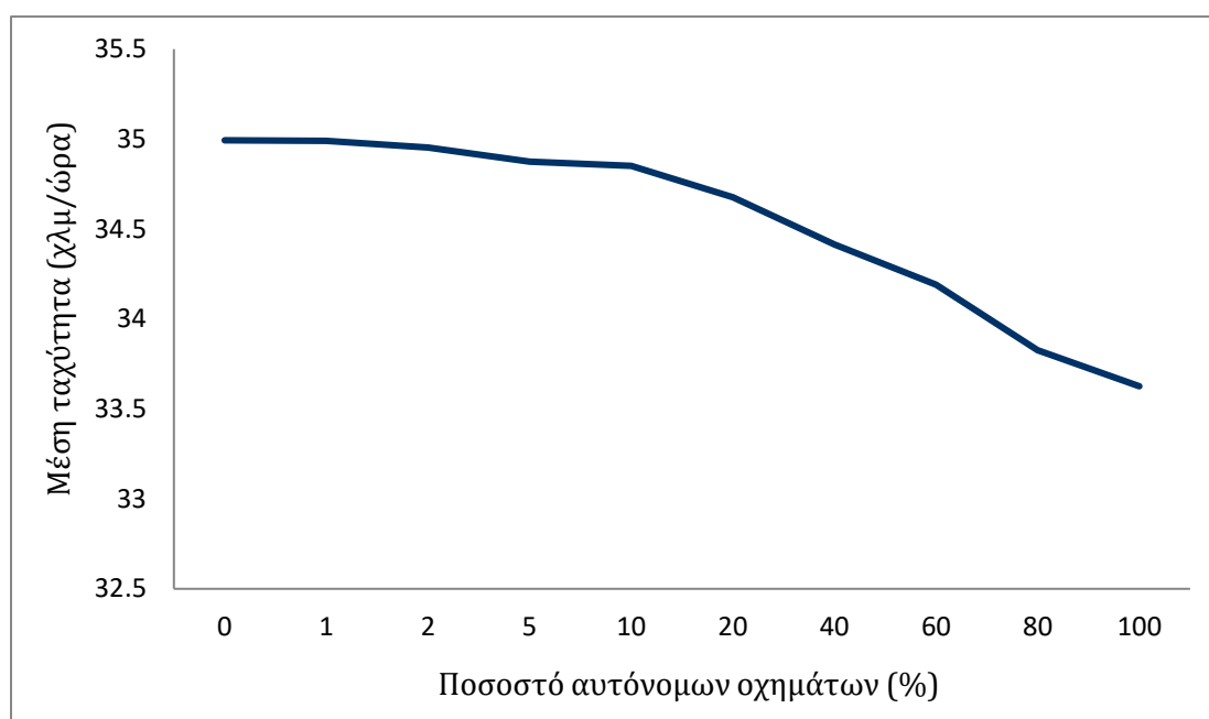
Διάγραμμα 5.2: Μέση ταχύτητα σε σχέση με το ποσοστό αυτόνομων οχημάτων στην κυκλοφορία.
