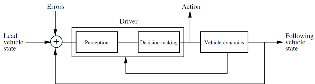
Εικόνα 3.1: Γενικό διάγραμμα αναπαράστασης μοντέλου ακολουθούντος οχήματος (Πηγή: Härrä, 2010) .
