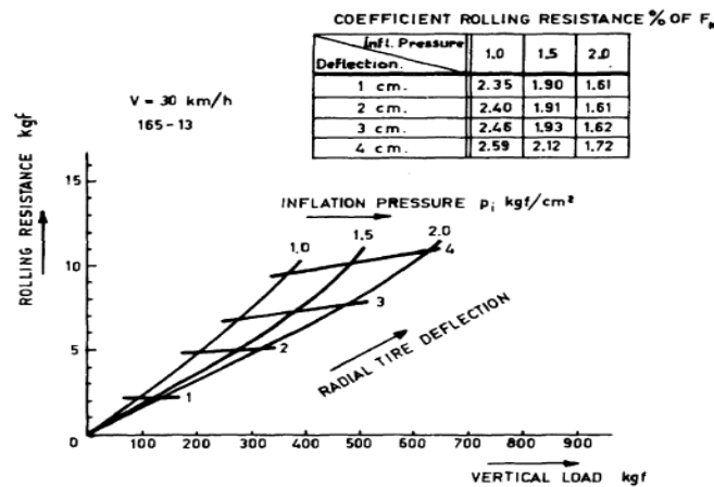
Εικόνα 2.7-Αντίσταση κύλισης συναρτήσει του φορτίου και της πίεσης του ελαστικού Πηγή: (Clark, 1971)
