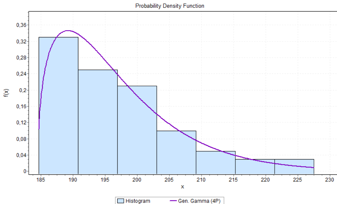
Εικόνα 4.4-Κατανομή συχνοτήτων αντίστασης κύλισης του δεδομένου τμήματος με τον αλγόριθμο N3
