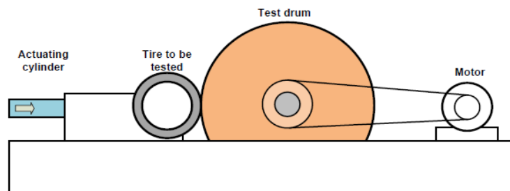
Εικόνα 3.1-Τυπική διάταξη της μεθόδου μέτρησης με τύμπανο Πηγή: (Sandberg, et al., 2011)
