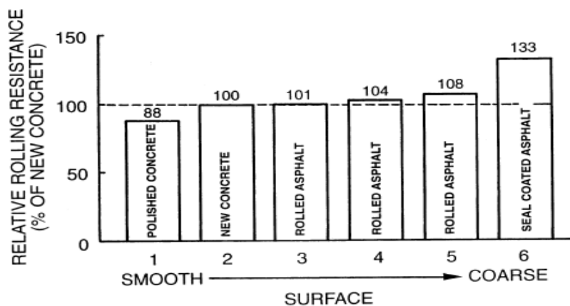
Εικόνα 2.18-Επιρροή της επιφάνειας του οδοστρώματος στην αντίσταση κύλισης Πηγή: (Clark, 1971)
