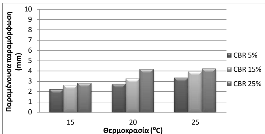
Εικόνα 5.48: Διάγραμμα μεταβολής παραμενουσών παραμορφώσεων διατομών Y1, Y2, Y3 ( V=100\text{km/h} )
