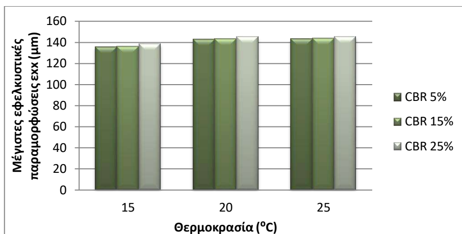
Εικόνα 5.27: Διάγραμμα μεταβολής μέγιστων εφελκυστικών παραμορφώσεων διατομών X1, X2, X3 ( V=60\text{km/h} )
