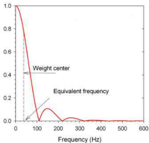
Εικόνα 3.9: Διάγραμμα ανηγμένης παραμόρφωσης συναρτήσει της συχνότητας (Πηγή: (Ghanizadeh & Fakhri, 2017))
