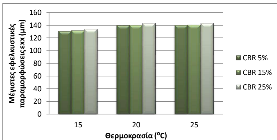
Εικόνα 5.28: Διάγραμμα μεταβολής μέγιστων εφελκυστικών παραμορφώσεων διατομών X1, X2, X3 ( V=100\text{km/h} )
