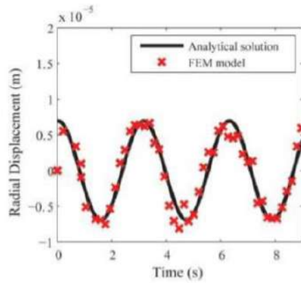
Εικόνα 3.8: Διάγραμμα υποχώρησης συναρτήσει του χρόνου φόρτισης (Πηγή: (Khavasefat, Jelagin, & Birgisson, 2014))
