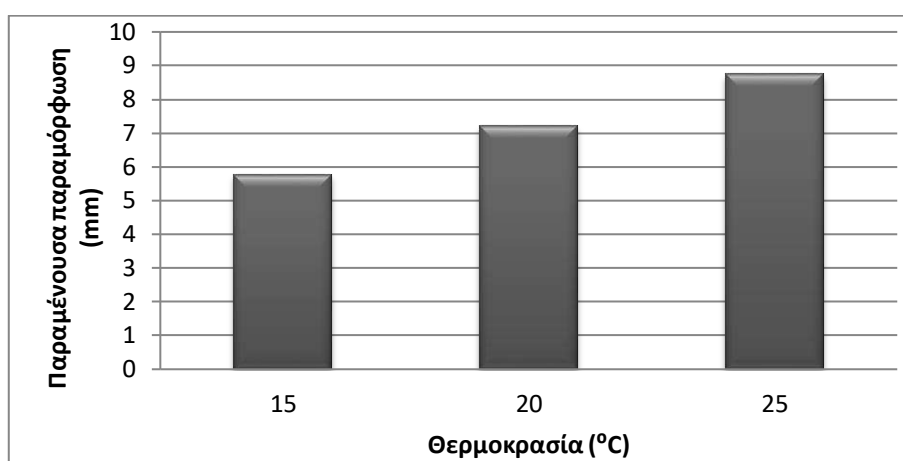
Εικόνα 5.7: Διάγραμμα παραμένουσας παραμόρφωσης-θερμοκρασίας διατομής Χ1 (V=60km/h)
