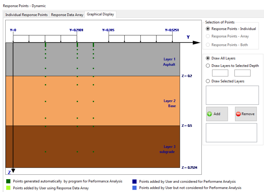
Εικόνα 4.7: Γραφική απεικόνιση σημείων απόκρισης (Πηγή:(Seyyedmahdi, 2015))
