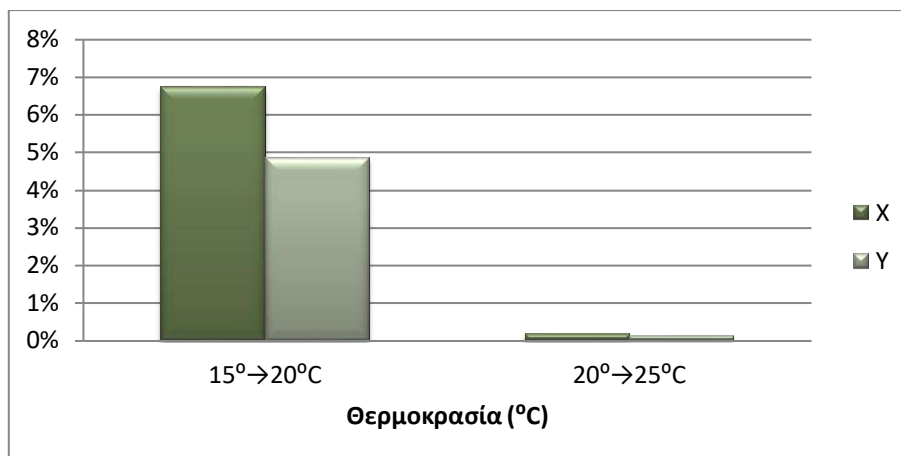
Εικόνα 5.54: Διάγραμμα ποσοστιαίας μεταβολής μέγιστων εφελκυστικών παραμορφώσεων ( V=100\text{km/h} )
