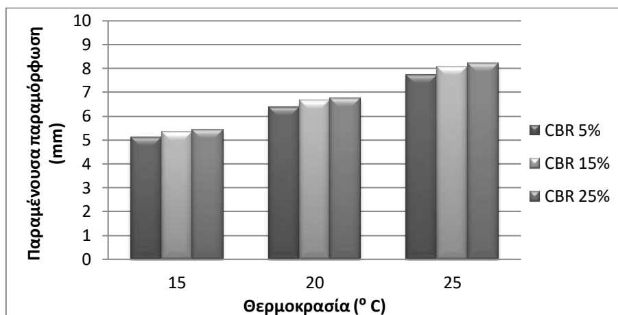
Εικόνα 5.26: Διάγραμμα μεταβολής παραμενουσών παραμορφώσεων διατομών X1, X2, X3 (V=100km/h)
