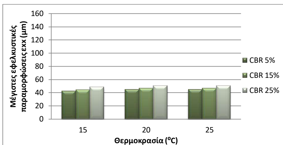
Εικόνα 5.50: Διάγραμμα μεταβολής μέγιστων εφελκυστικών παραμορφώσεων διατομών Υ1, Υ2, Υ3 (V=100km/h)
