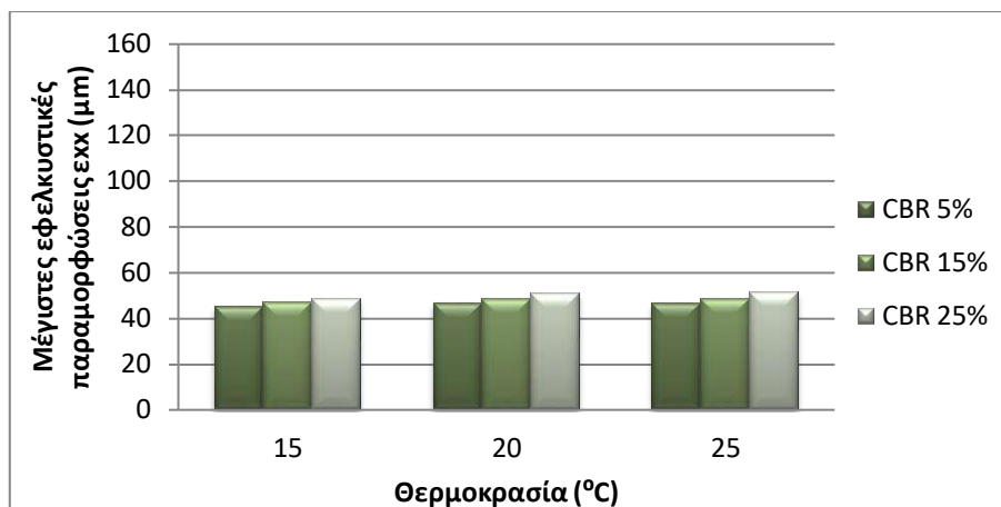
Εικόνα 5.49: Διάγραμμα μεταβολής μέγιστων εφελκυστικών παραμορφώσεων διατομών Υ1, Υ2, Υ3 (V=60km/h)
