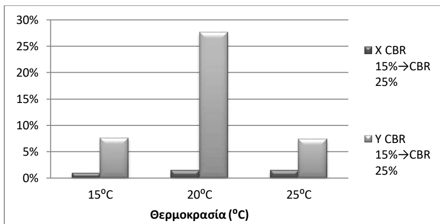
Εικόνα 5.60: Διάγραμμα ποσοστιαίας μεταβολής παραμενουσών παραμορφώσεων με αύξηση δείκτη CBR (V=100km/h)
