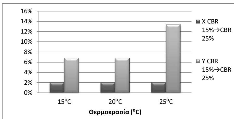
Εικόνα 5.59: Διάγραμμα ποσοστιαίας μεταβολής παραμενουσών παραμορφώσεων με αύξηση δείκτη CBR (V=60km/h)
