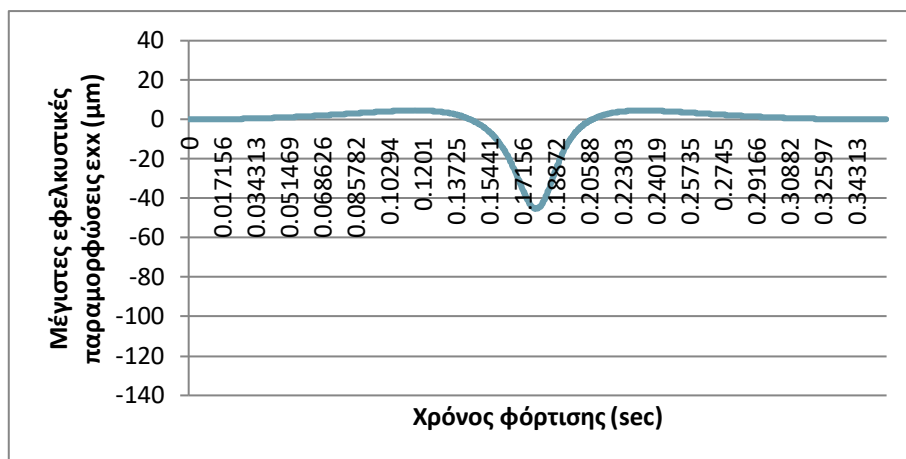
Εικόνα 5.6: Τυπική κατανομή εφελκυστικής παραμόρφωσης ενδιάμεσα των δύο τροχών σε διατομή υψηλού κυκλοφοριακού φόρτου.
