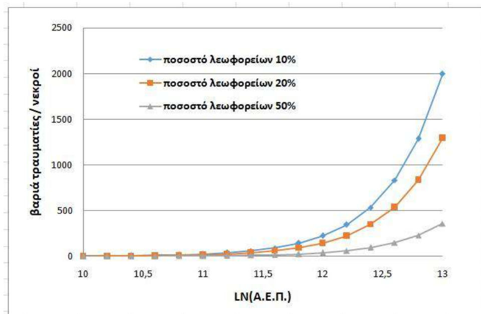
Διάγραμμα 5.10 : Διάγραμμα ευαισθησίας για την επιρροή του ποσοστού των λεωφορείων στη σοβαρότητα των οδικών ατυχημάτων.
