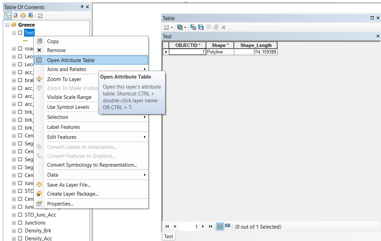
Εικόνα 5.9 Attribute Table
