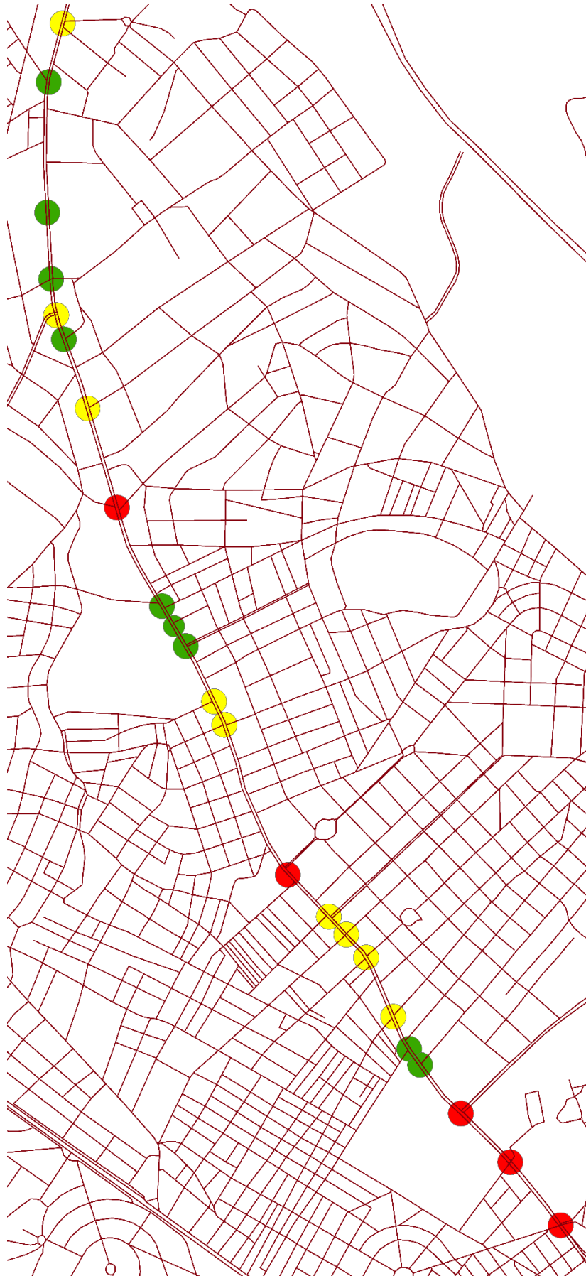
Χάρτης 5.9 Πιθανότητα απότομης επιτάχυνσης σε κόμβο χρωματικά
