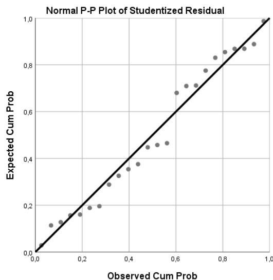
Διάγραμμα 6.3 Αθροιστική πιθανότητα σφάλματος για το μοντέλο επιταχύνσεων ανά ημέρα σε κόμβο
