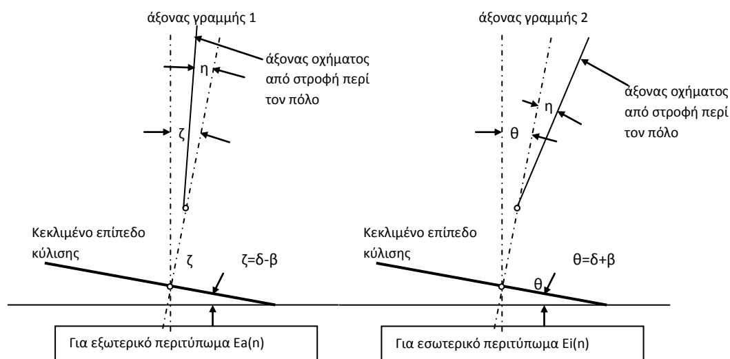
Σχήμα 4.10: Δυσμενέστερη θέση περιτυπωμάτων που καθορίζει την απόσταση στο εσωράχιο της σήραγγας στην καμπύλη
