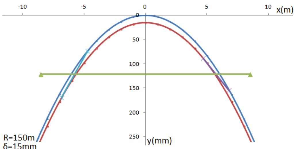
Σχήμα 3.13: Vogelplan οχημάτων Μετρό για R=150\text{m} με διαπλάτυνση 5\text{mm}
