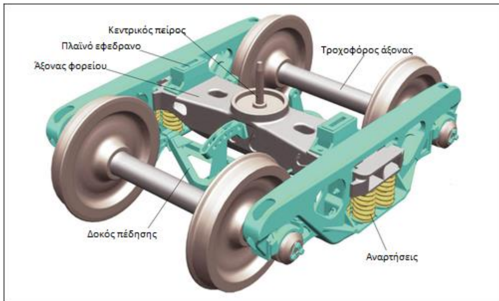
Εικόνα 2.2: Διαξονικό φορείο
