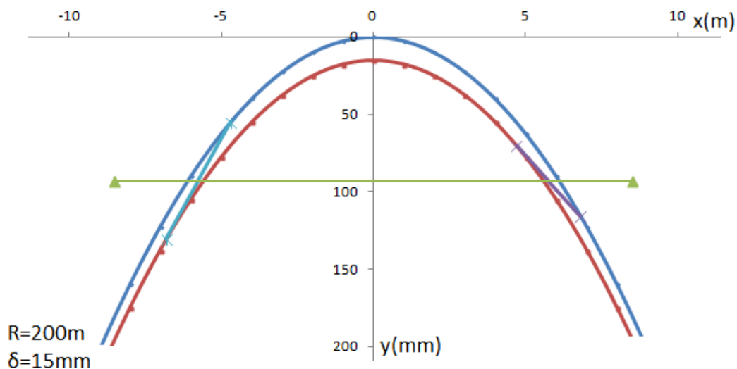
Σχήμα 3.12: Vogelplan οχημάτων Μετρό για R=200\text{m} με διαπλάτυνση 5\text{mm}
