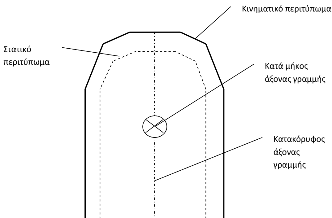
Σχήμα 4.2: Διατομή γραμμής με το στατικό και το κινηματικό περιτύπωμα
