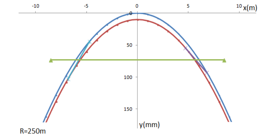
Σχήμα 3.10: Vogelplan οχημάτων Μετρό για R=250m
