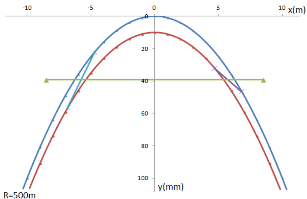
Σχήμα 3.6: Vogelplan οχημάτων Μετρό για R=500\text{m}
