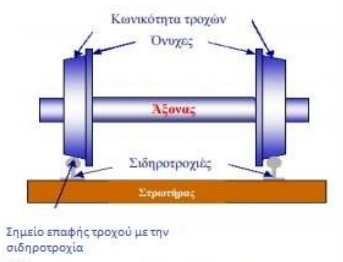
Εικόνα 2.1: Σύστημα τροχών - Σιδηροτροχιάς
