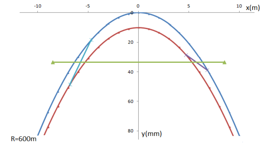
Σχήμα 3.5: Vogelplan οχημάτων Μετρό για R=600m
