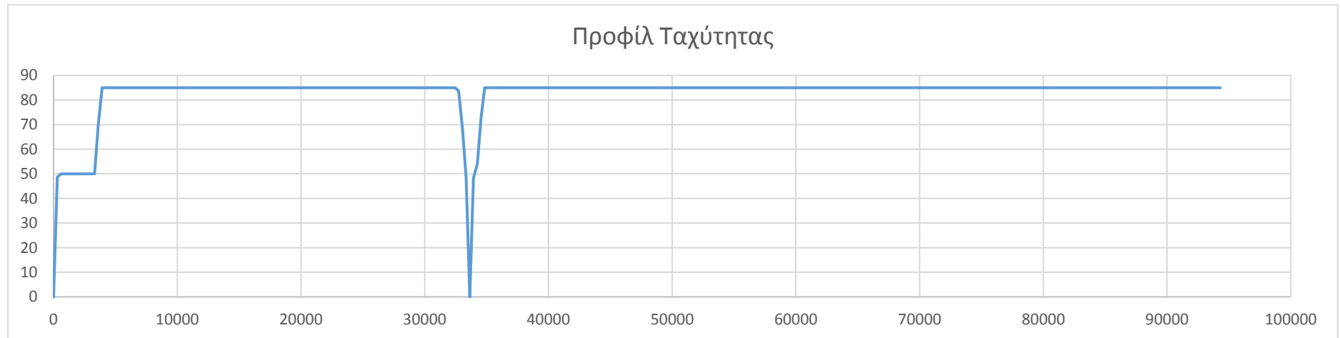
Διάγραμμα 4: Προφίλ ταχύτητας για τη διαδρομή Πειραιάς-Θήβα μέσω εθνικής
