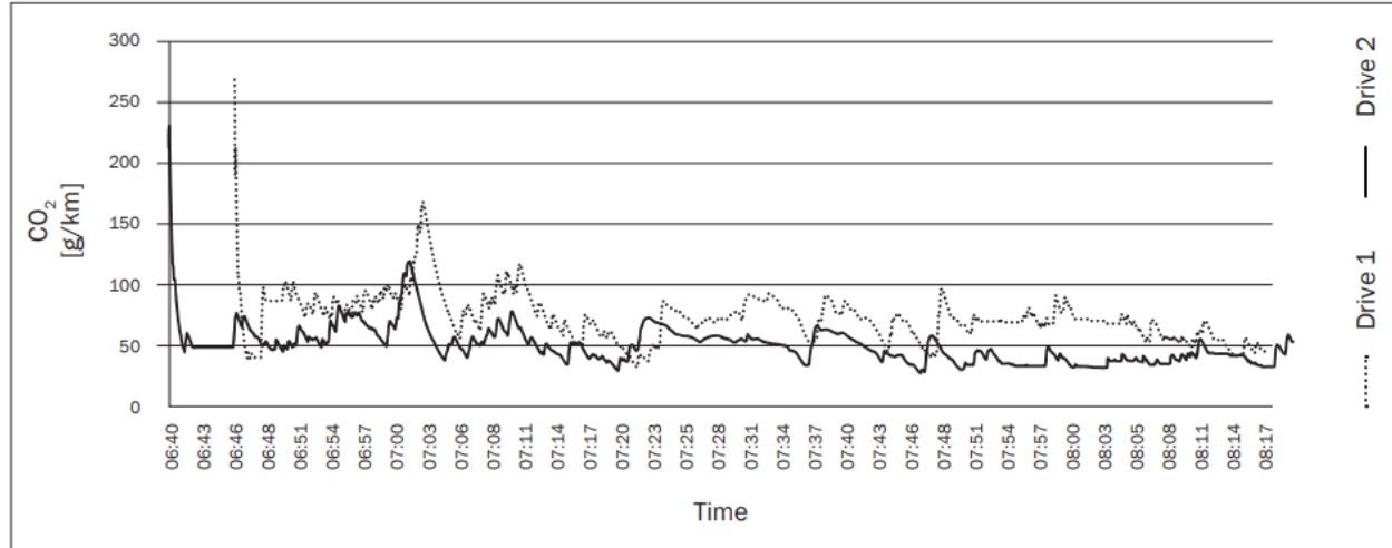
Διάγραμμα 7: Σύγκριση εκπομπών CO 2 κατά την κανονική οδήγηση και κατά το eco-driving. Πηγή: [34]
