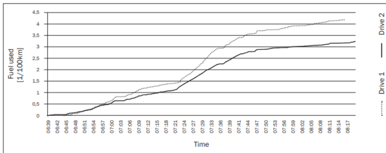
Διάγραμμα 6: Σύγκριση κατανάλωσης καυσίμου κατά την κανονική οδήγηση και κατά το eco-driving. Πηγή: [34]
